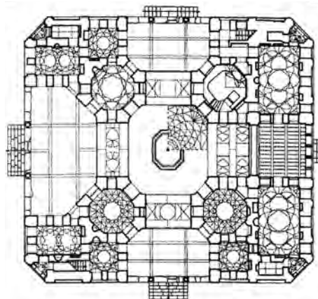
پلان طبقه اول
